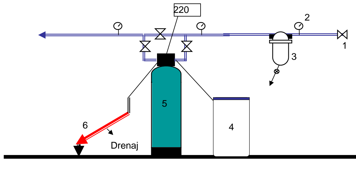
Schemă de montaj
